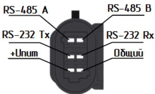
Рисунок 7. Разъем БИС 20240 для подключения внешнего устройства
